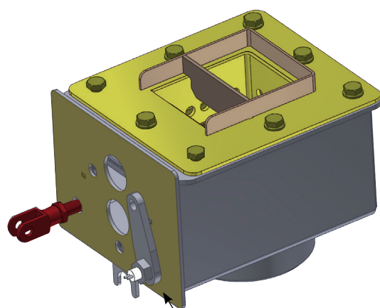
Elemento d'accensione
