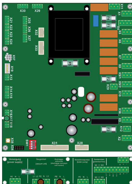
Allacciamento unità di aspirazione:
