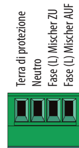
X 3 (gruppo di miscelazione)
