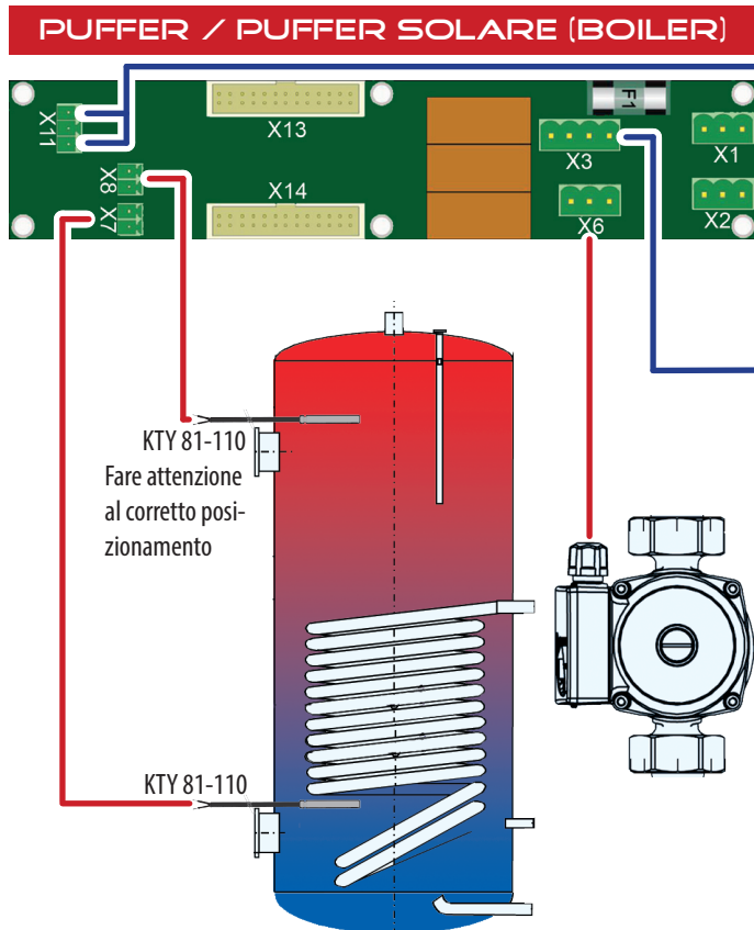
X 8 Sonda del puffer SOPRA X 7 (Sonda del puffer SOTTO)
