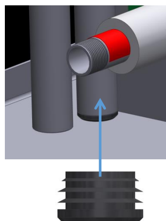
[2.1] Stopfen in Primärluftkanal einpressen
