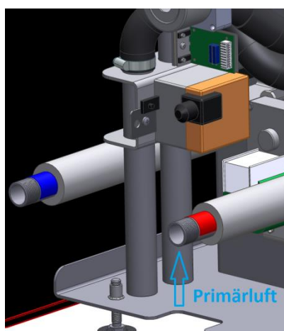
[2.0] Primärluft = hinteres Rohr mit LMS Sensor
