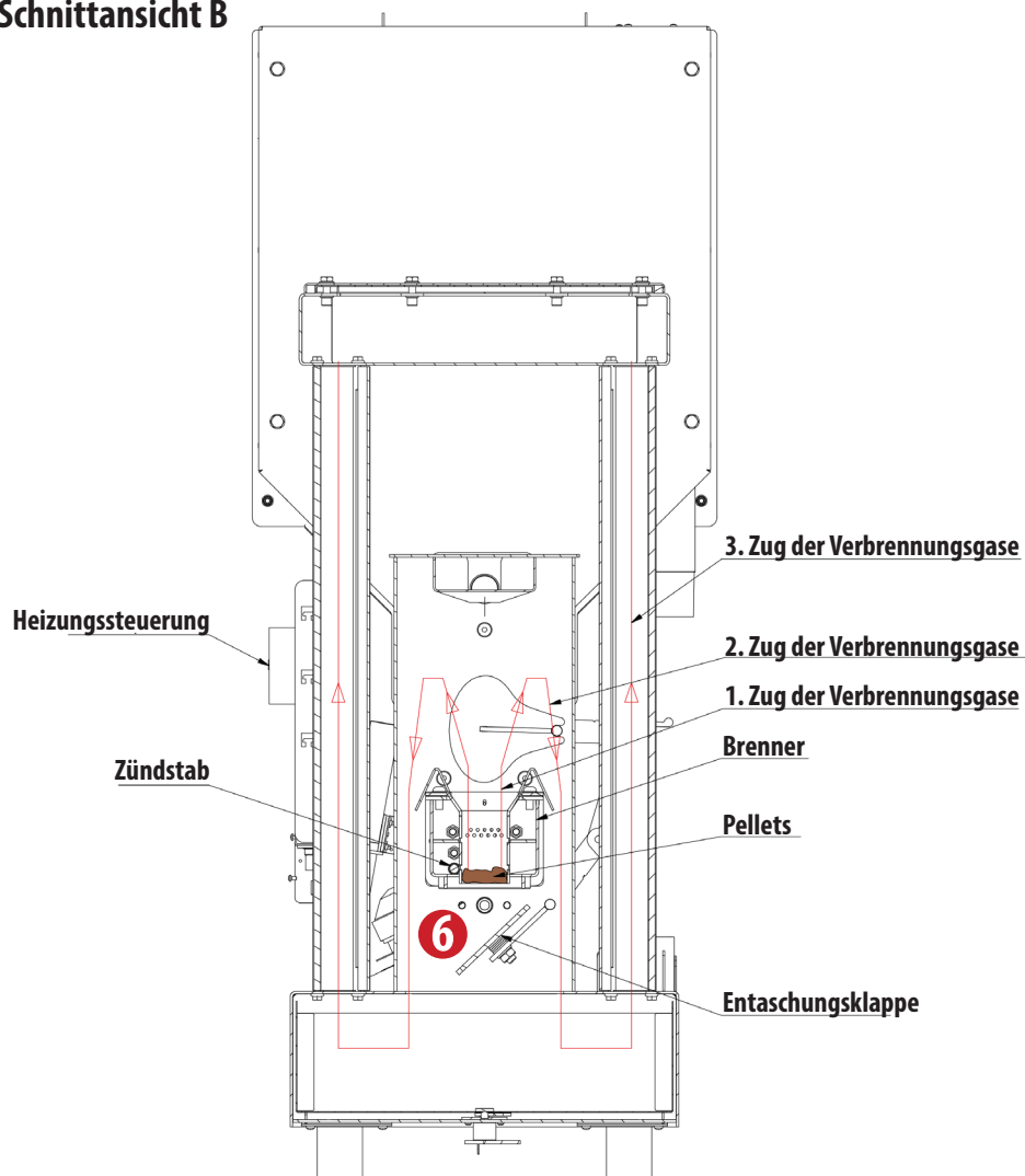
Schnittansicht B
